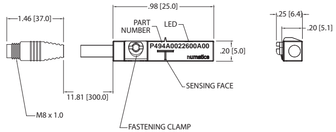
PNP-QDS-M8-U
